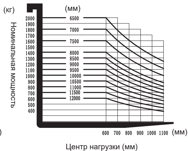
Диаграмма остаточной грузоподъемности
